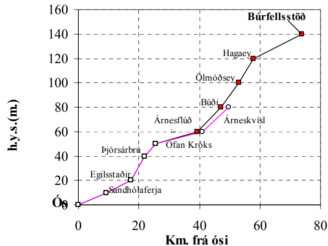
Mynd 5.2 Langsnið Þjórsár frá ósi að Búrfelli.
