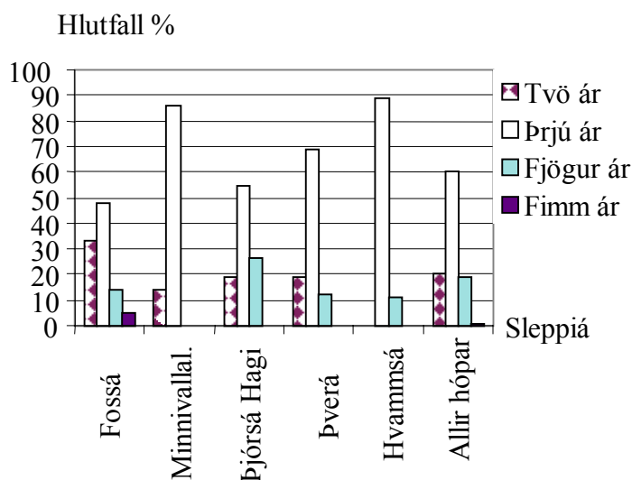
Mynd 9.5.2 Hlutfallsleg skipting heimta sumaralinna seiða eftir árum frá sleppingu, skipt eftir sleppiám.
