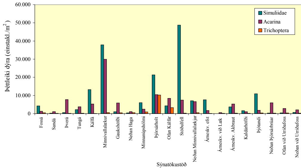
Mynd 9.2.5 Fjöldi bitmýslirfa (Simuliidae), vatnamaura (Acarina) og vorflugulirfa (Trichoptera) á vatnasviði Þjórsár. Sýnum úr þverám Þjórsár er raðað frá efstu til neðstu ár og úr Þjórsá frá efstu til neðstu stöðvar.
