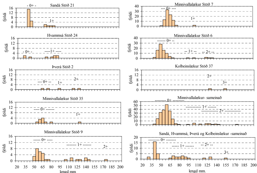
Mynd 9.4.3 Lengdar- og aldursdreifing laxa- og bleikjuseiða í þverám Þjórsár ofan Búða og Hestafoss. Úr seiðarannsóknum 2001. Sjá skýringar við mynd 9.4.2.
