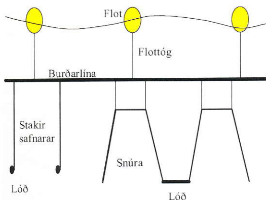
Mynd 2.10. Snúrur og stakir safnara.
