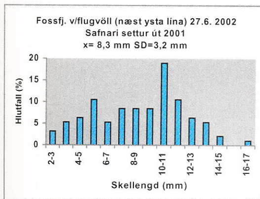
3. mynd. Lengdardreifing, meðallengd og staðalfrávik kræklinga á söfnurum v/flugvöll í Fossfirði í mars og júní 2002.
