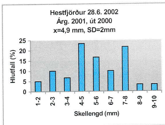
6. mynd. Lengdardreifing, meðallengd og staðalfrávik kræklinga á söfnurum í Hestfirði í júní 2002.
