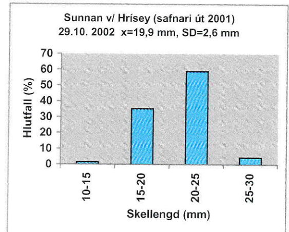
10. mynd. Lengdardreifing, meðallengd og staðalfrávik kræklinga á söfnurum frá 2001 og 2002 hjá Norðurskel sunnan v/ Hrísey í október 2002.
