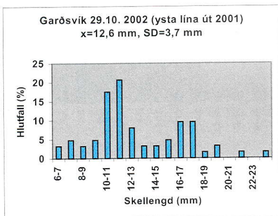
8. mynd. Lengdardreifing, meðallengd og staðalfrávik kræklinga á söfnurum hjá Marbendli í Garðsvík í október 2002.
