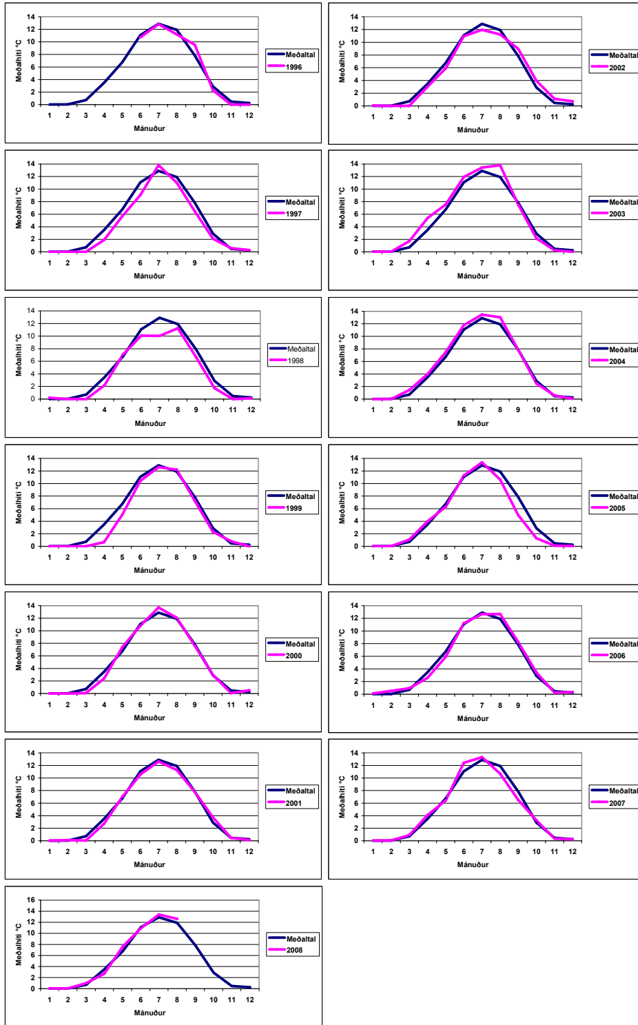
13. mynd. Vatnshiti í Laxá í Aðaldal, mælt með síritandi hitamæli við brú hjá Laxamýri 1996 til ágúst 2008. Hitaferlar einstakra ára eru bornir saman við meðalhita tímabilsins 1996-2005.
