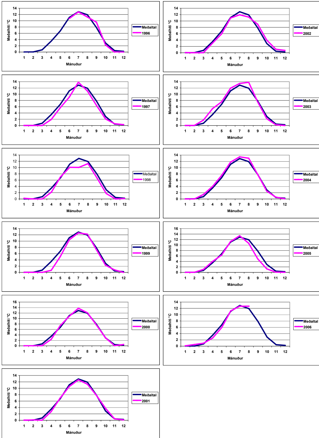
12. mynd. Vatnshiti í Laxá í Aðaldal, mælt með síritandi hitamæli við brú hjá Laxamýri 1996 til ágúst 2006. Hitaferlar einstakra ára eru bornir saman við meðalhita alls tímabilsins.
