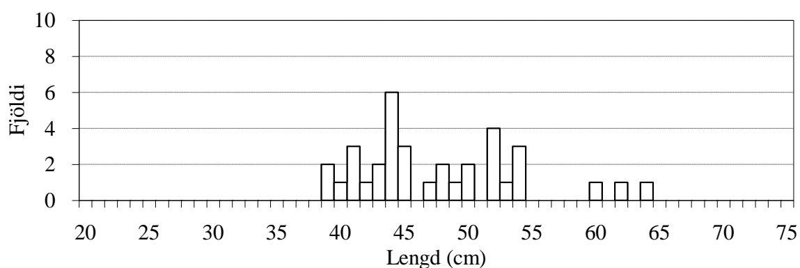
23. mynd. Lengdardreifing aldursgreindra urriða úr Þjórsá árið 2006.
