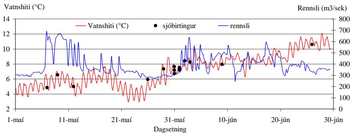
14. mynd. Vatnshiti og rennsli Þjórsár og ganga útvarpsmerktra sjóbirtinga niður fyrir gömlu Þjórsárbrú vorið 2006.
