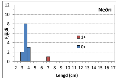
6. mynd. Lengd og aldur lax, bleikju og urriða sem veiddist í rafveiði í Gilsá í ágúst 2014.
