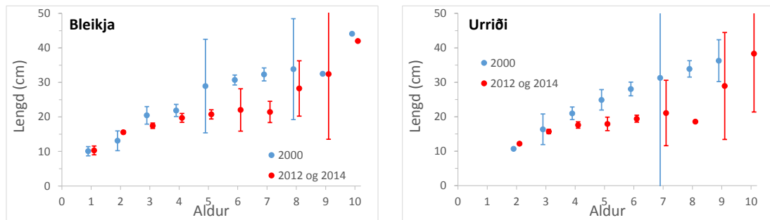
29. mynd. Meðallengd (með 95% öryggismörkum) árganga bleikju og urriða sem veiddust í Vífilsstaðaflóa fyrir (2000) og eftir (2012 og 2014) Kárahnjúkavirkjun.
