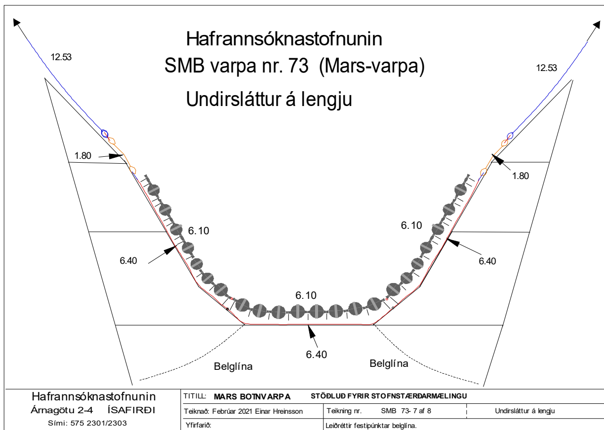
Mars botnvarpa nr. 73. Undirsláttur á lengju.
