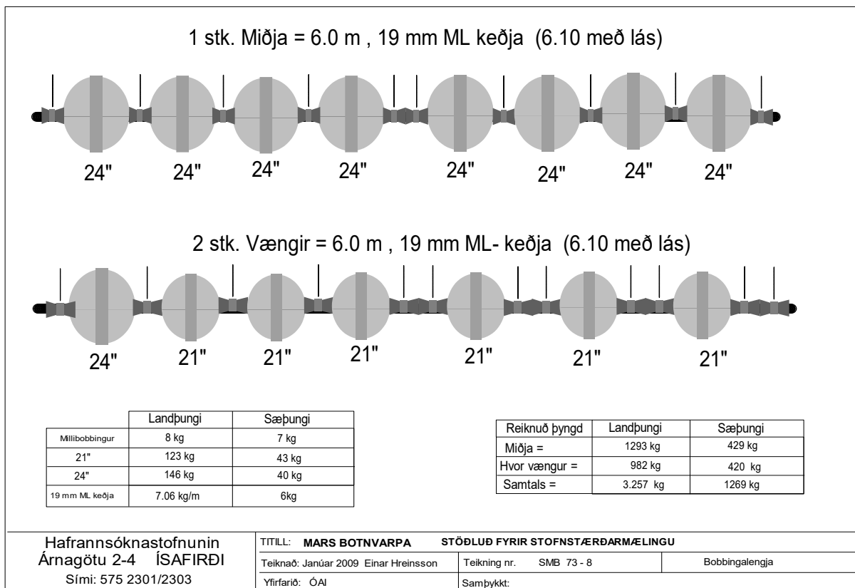
Mars botnvarpa nr. 73. Bobbingalengja.
