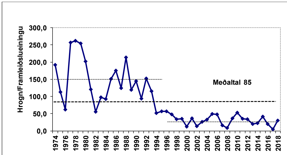
9. mynd. Áætlaður fjöldi hrogn á hverja framleiðslueiningu í Reykjadalsá á árunum 1974 - 2018 (meðaltal 1974 - 1993 er 150 og meðaltal 1994 - 2018 er 33) (mat á fjölda framleiðslueininga byggir á bráðabirgðamati).
