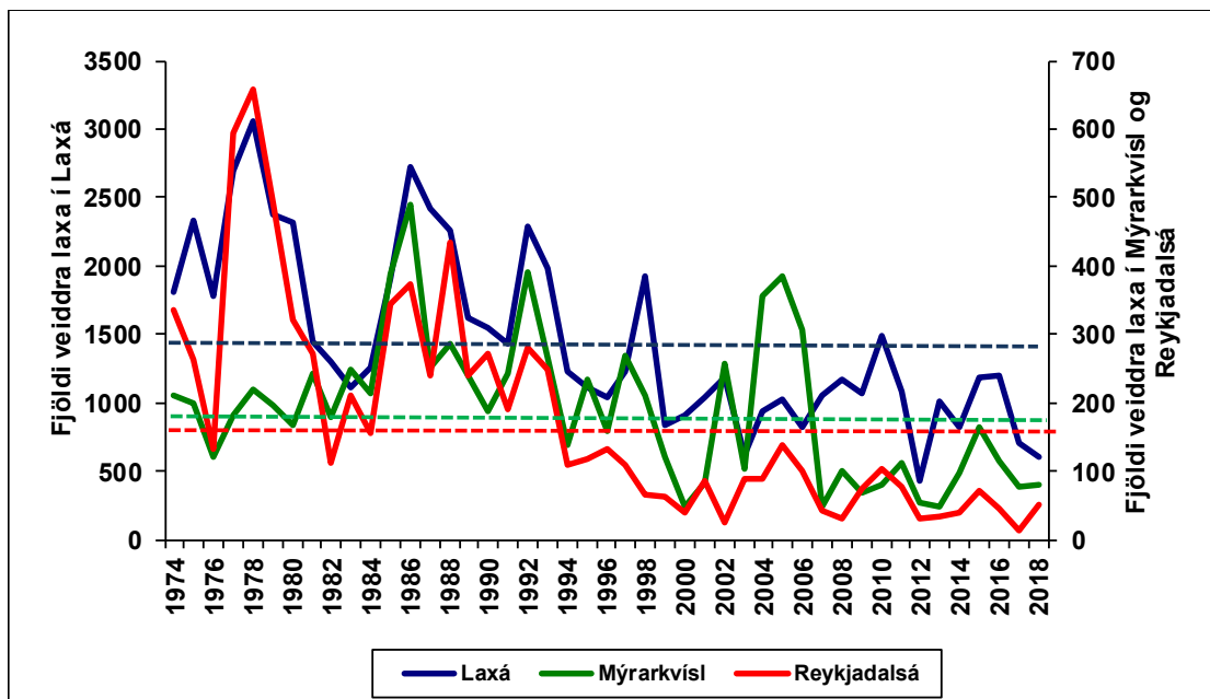
6. mynd. Skráð laxveiði á stöng í Laxá í Aðaldal, Mýrarkvísl og Reykjadalsá og Eyvindarlæk á árunum 1974 - 2018. Sá lax sem sleppt er aftur er með í þessum tölum. Brotnar línur sýna meðaltöl.
