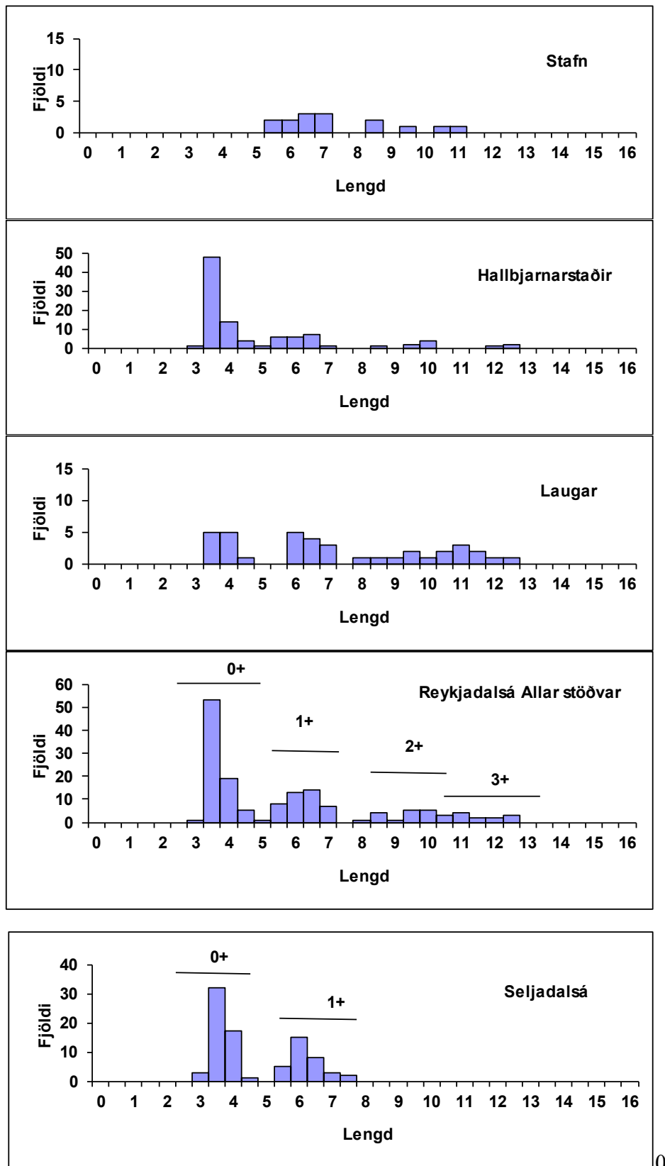
1. mynd. Lengdardreifing laxaseiða í rafveiðum í Reykjadalur og Seljadalsá sumarið 2018.
