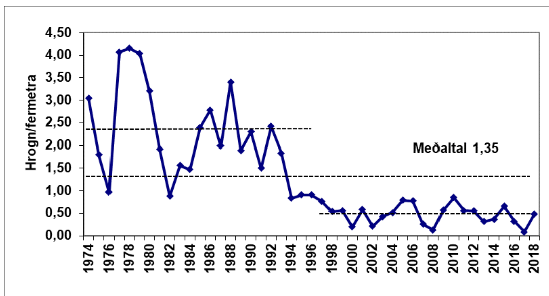
8. mynd. Áætlaður fjöldi hrogna á hvern fermetra botnflatar í Reykjadalsá á árunum 1974 - 2018 (meðaltal 1974-1993 er 2,38 og meðaltal 1994 - 2018 er 0,53).
