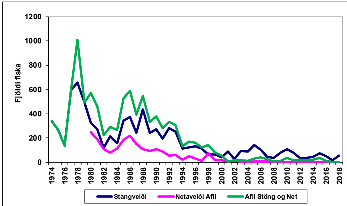
5. mynd. Stangveiði, netaveiði og afli (fjöldi landaðra laxa) á vatnasvæði Reykjadalsár og Eyvindarlækjar 1974 - 2018.
