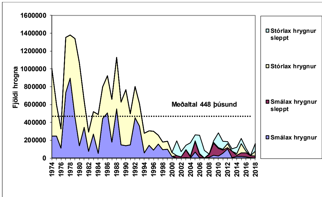
7. mynd. Áætlaður fjöldi hrogna í hrygningu í Reykjadalsá og Eyvindarlæk. Gert er ráð fyrir að veiðihlutfall í stangveiði hafi verið 50% á smálax og 70% á stórlax, kynjahlutfall í veiði og hrygningu hafi verið það sama og tekið tillit til stærðar hrygna. Gert er ráð fyrir að 30% þeirra fiska sem sleppt var hafi verið sleppt einu sinni eða oftár.
