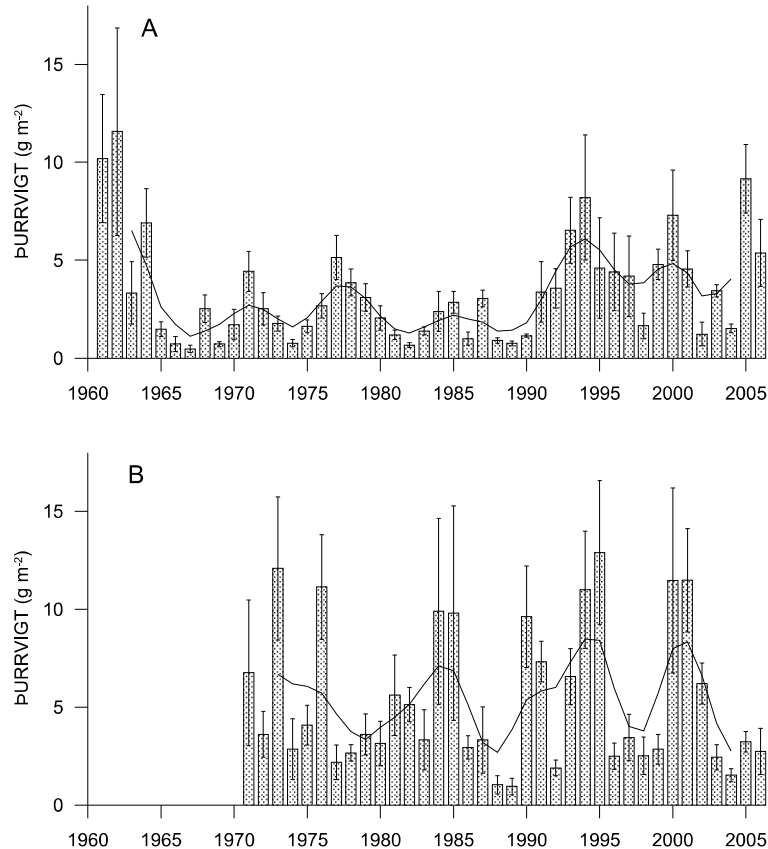
10. mynd. Breytingar á átumagni ( \text{g þurrvigt m}^{-2} , 0-50 m) að vorlagi á A) Siglunessniði, og B) Selvogsbankasniði. Súlnurnar sýna meðaltöl allra stöðva á sniðinu. Staðalskekkja er sýnd með lóðréttum strikum. Einnig er sýndur reiknaður ferill (5 ára keðjumeðaltöl) sem jafnar miklar óreglur einstakra ára. Lega rannsóknasniðanna er sýnd á 1 mynd.
