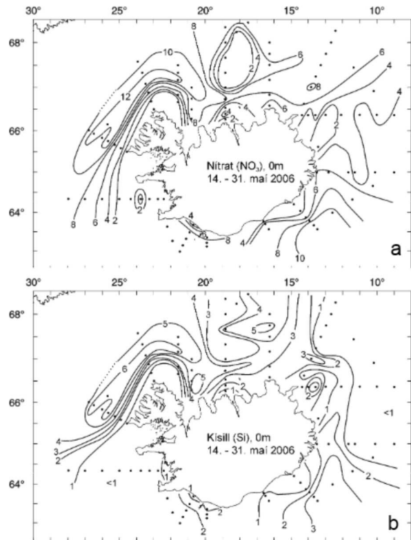
4. mynd. Styrkur næringarefna við yfirborð í hafinu umhverfis Ísland 14.–31. maí 2006, a) níturat ( \text{NO}_3 , \mu\text{mol l}^{-1} ) og b) kísill ( \text{Si} , \mu\text{mol l}^{-1} ).
