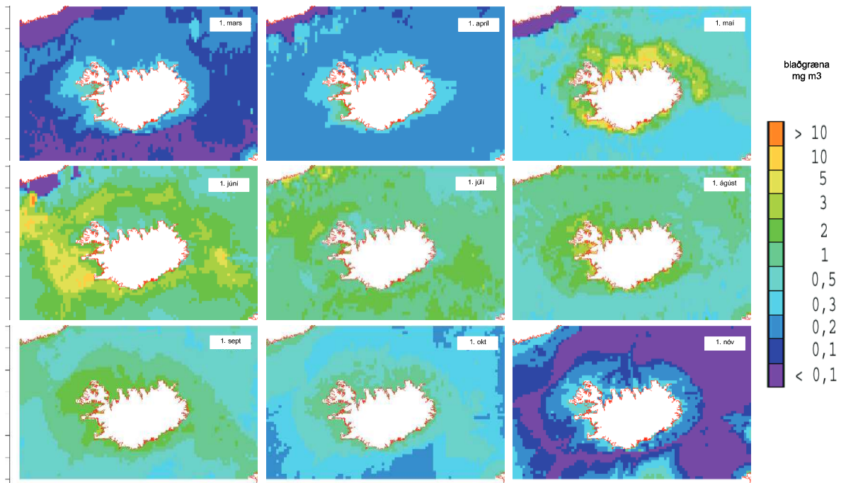
26. mynd. Lárétt dreifing blaðgrænu (mg m-3), fyrsta dag hvers mánaðar frá mars til nóvember, samkvæmt tölfraðilegu líkani af framvindu gróðurs við yfirborðið á hafsvæðinu umhverfis Ísland.
