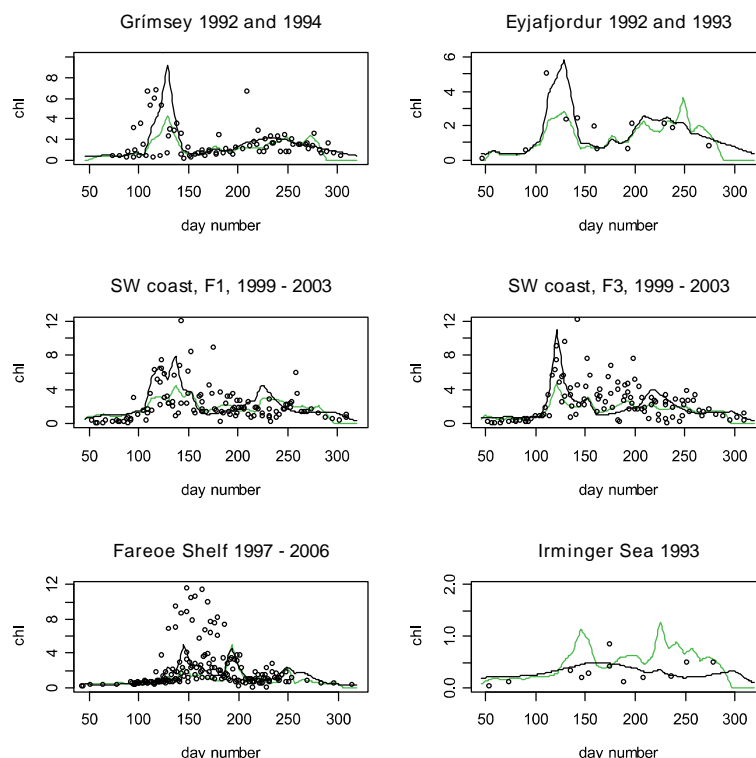
27. mynd. Ársferlar sem sýna breytingar í magni blaðgrænu ( \text{mg m}^{-3} ) á sex völdum stöðvum, þar sem reglubundnar mælingar á sjósýnum eru fyrirleggjandi. Myndirnar sýna niðurstöður mælinga á sjósýnum (deplar), staðlaðar niðurstöður NASA á magni blaðgrænu við yfirborð sjávar samkvæmt mælingum frá gervihnetti, SeaWiFS (grænn ferill) og leiðrétt blaðgrænu gildi samkvæmt tölfræðilíkani í umræddri rannsókn (svartur ferill).
