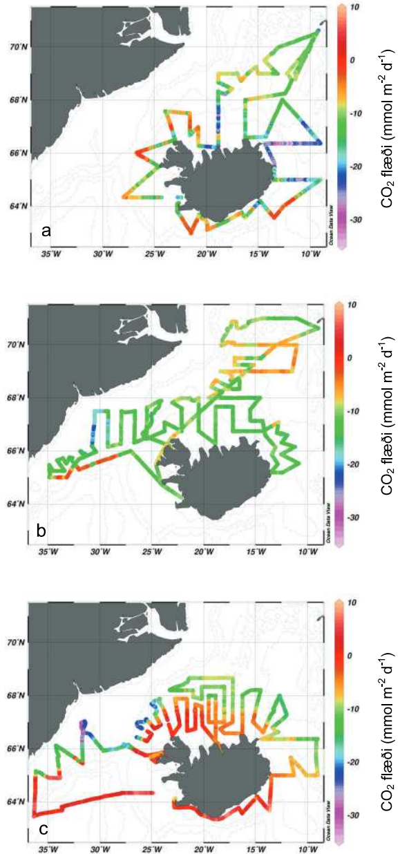
28. mynd. Flæði koldíoxíðs milli sjávar og loftis árið 2006 í a) maí, b) júlí og c) nóvember. Koldíoxíð flæðir frá sjó til loftis þegar gildin eru pósitíf, en flæðið er frá lofti til sjávar þegar gildin eru neikvæð.
