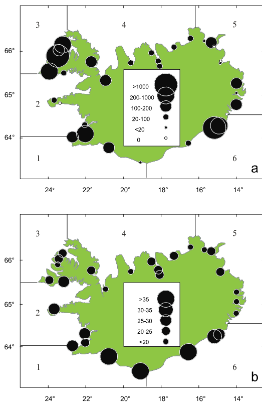
21. mynd. Þéttleiki (einstaklingar 100 m -2 ) a) og meðallengd (mm) b) skarkolaseiða ( Pleuronectes platessa ) í synatökum við Ísland síðari hluta júlímánaðar 2006. Tölurnar sýna skiptingu landgrunnans í svæði.
