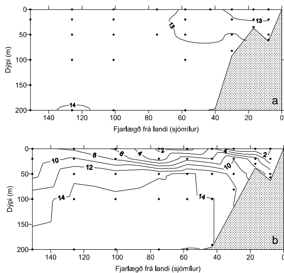
3. mynd. Lóðrétt dreifing nitrats ( \mu\text{mol l}^{-1} ) á Faxaflóasniði a) 1. – 2. febrúar 2006 og b) 14. maí 2006.
