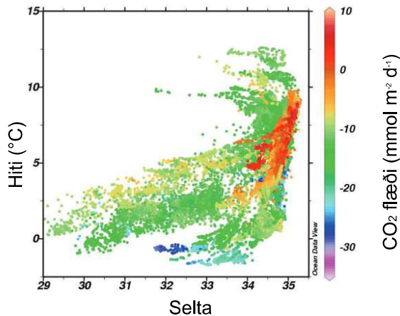
29. mynd. Hita-seltu línurit af yfirborðssjó úr leiðingrunum þremur. Litur punktanna segir til um flæði koldíoxíðs frá sjó til loftis.
