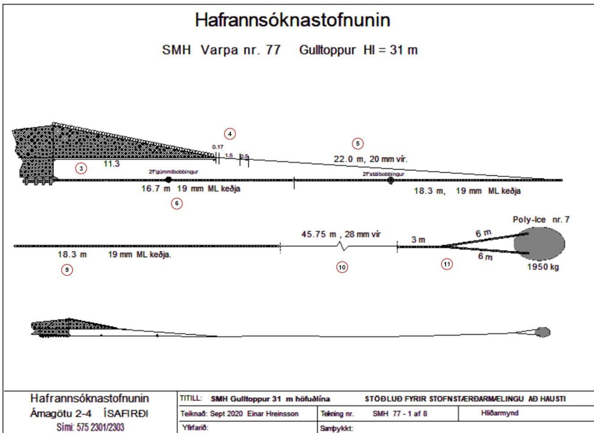
6. mynd. Gulltoppur, botnvarpa nr. 77, stöðluð fyrir Stofnmælingu botnfiska að haustlagi á grunnslóð. Hliðarmynd (miðnet að rossi).
