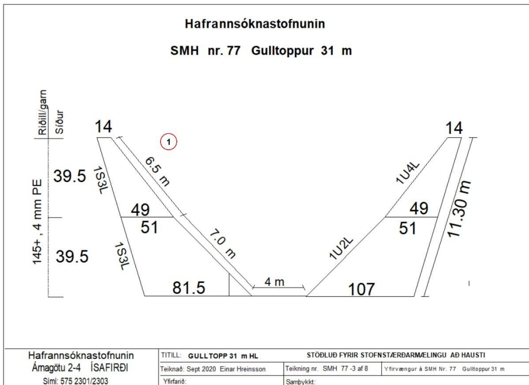
7. mynd. Gulltoppur, botnvarpa nr. 77, stöðluð fyrir Stofnmælingu botnfiska að haustlagi á grunnslóð. Yfirvængur.
