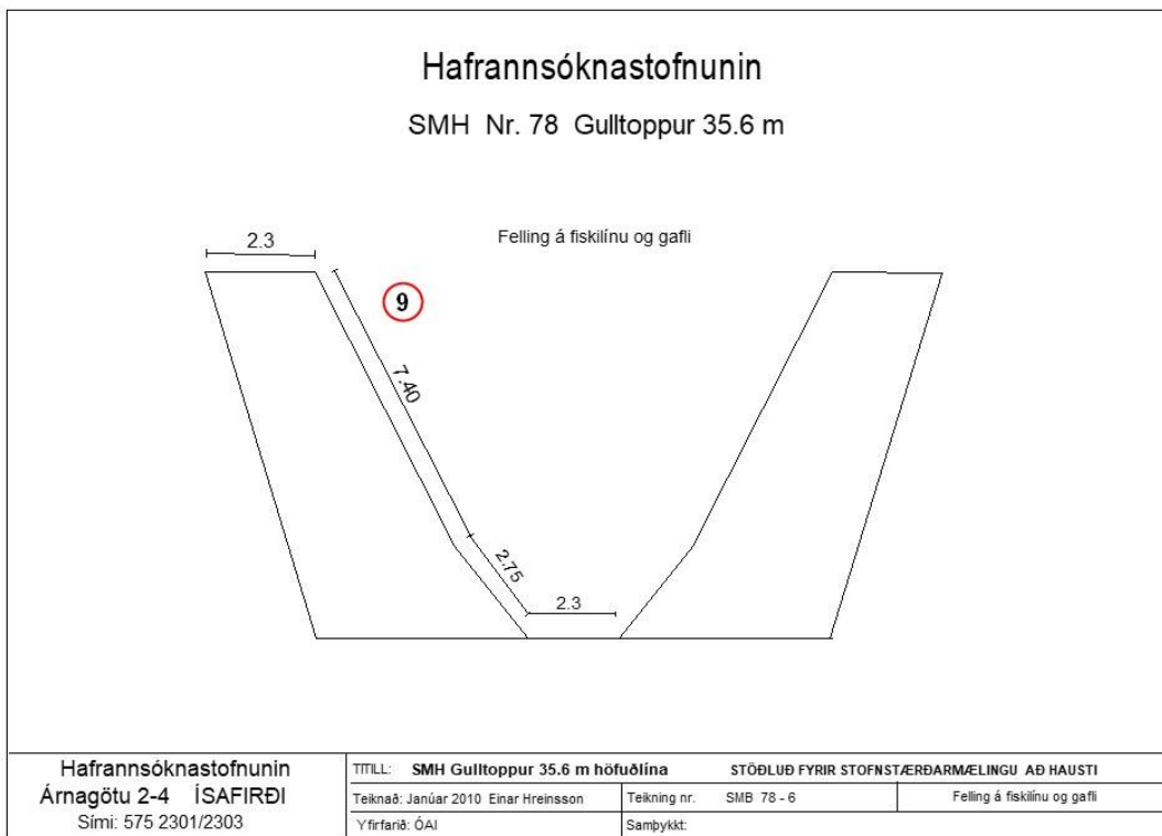
18. mynd. Gulltoppur, botnvarpa nr. 78, stöðluð fyrir Stofnmælingu botnfiska að haustlagi á djúpslóð. Felling á fiskilínu og gaffli.
