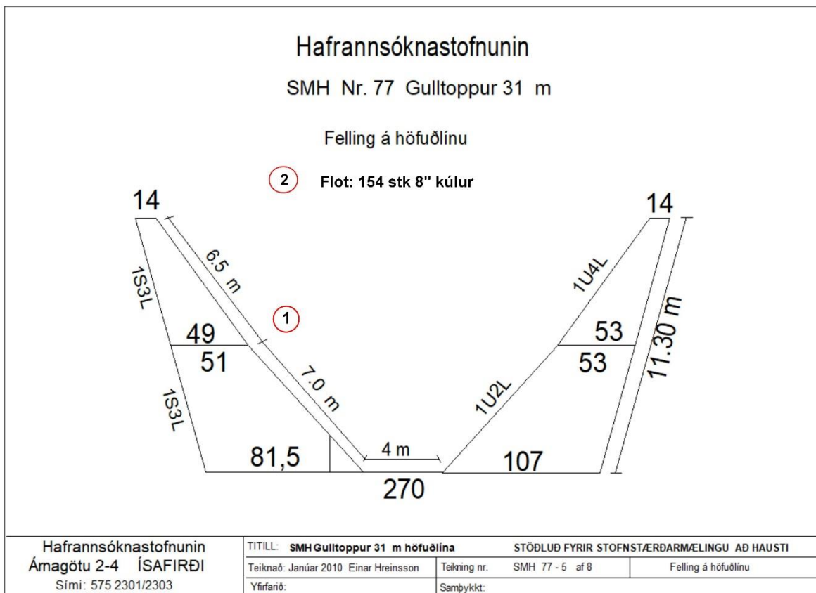
9. mynd. Gulltoppur, botnvarpa nr. 77, stöðluð fyrir Stofnmælingu botnfiska að haustlagi á grunnslóð. Felling á höfuðlinu.
