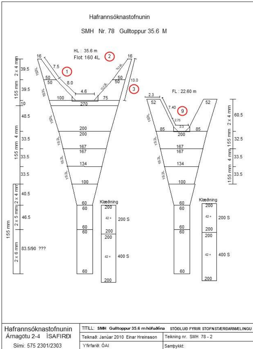
14. mynd. Gulltoppur, botnvarpa nr. 78, stöðluð fyrir Stofnmælingu botnfiska að haustlagi á djúpslóð. Yfirlitsmynd.
