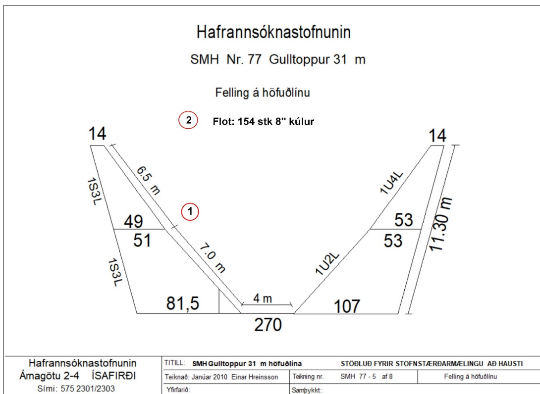
9. mynd. Gulltoppur, botnvarpa nr. 77, stöðluð fyrir Stofnmælingu botnfiska að haustlagi á grunnslóð. Felling á höfuðlínu.
