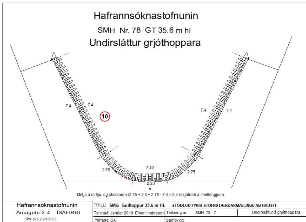
19. mynd. Gulltoppur, botnvarpa nr. 78, stöðluð fyrir Stofnmælingu botnfiska að haustlagi á djúpslóð. Undirsláttur grjóthoppa.
