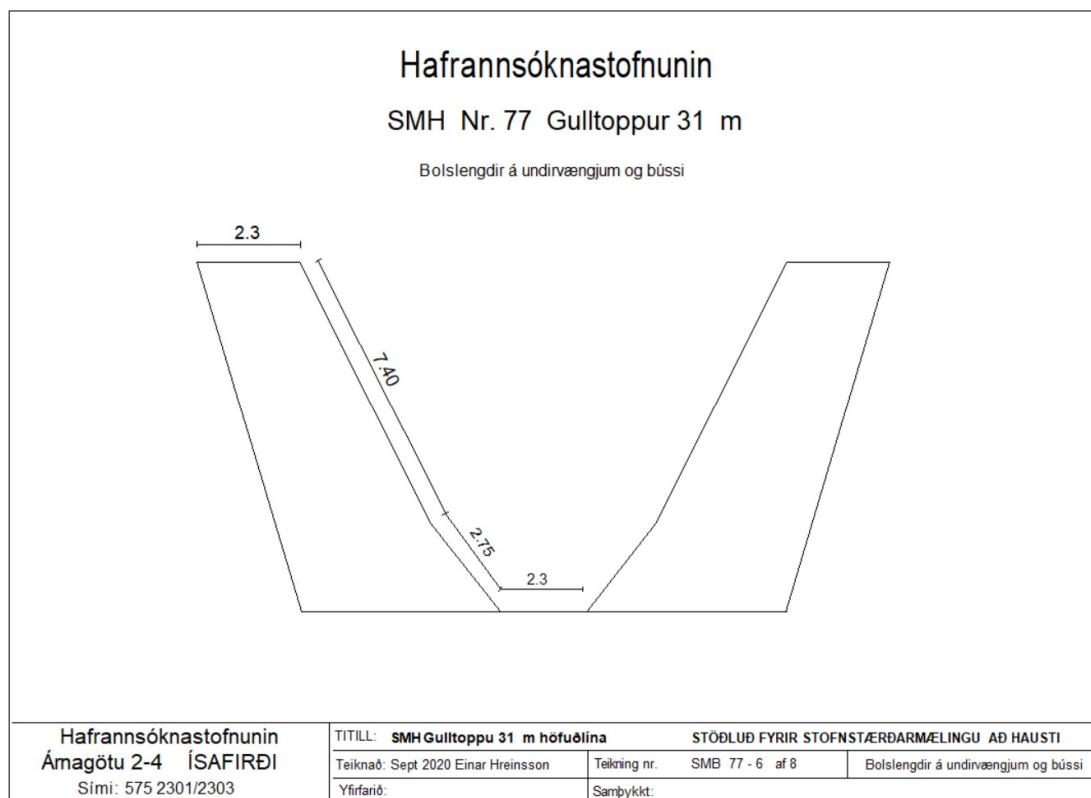
10. mynd. Gulltoppur, botnvarpa nr. 77, stöðluð fyrir Stofnmælingu botnfiska að haustlagi á grunnslóð. Felling á fiskilínu og afli.
