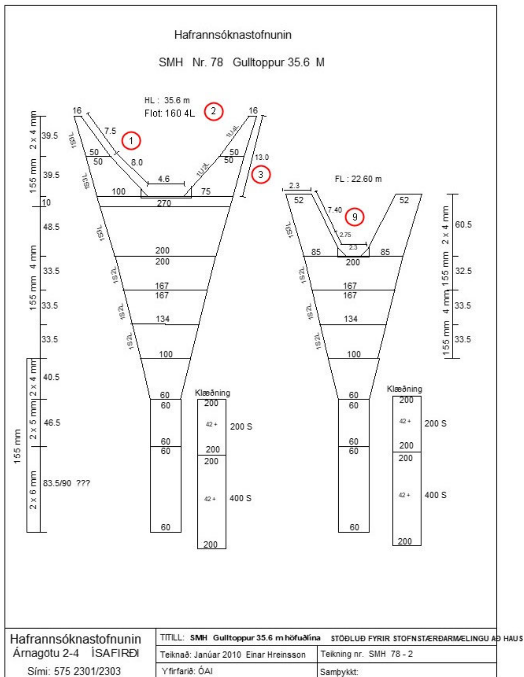
14. mynd. Gulltoppur, botnvarpa nr. 78, stöðluð fyrir Stofnmælingu botnfiska að haustlagi á djúpslóð. Yfirlitsmynd.
