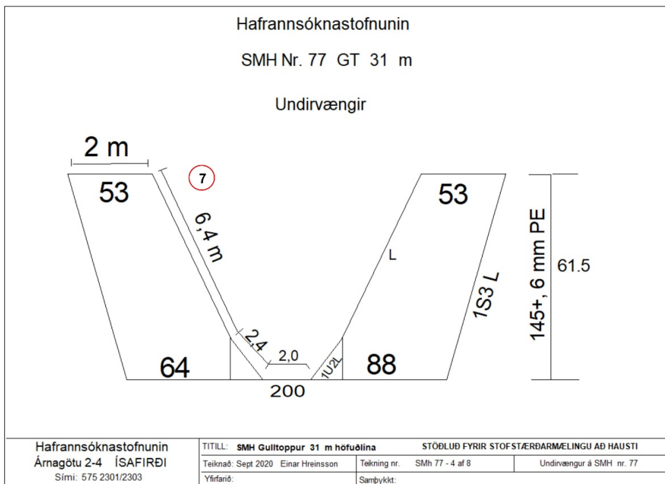
8. mynd. Gulltoppur, botnvarpa nr. 77, stöðluð fyrir Stofnmælingu botnfiska að haustlagi á grunnslóð. Undirvængur.
