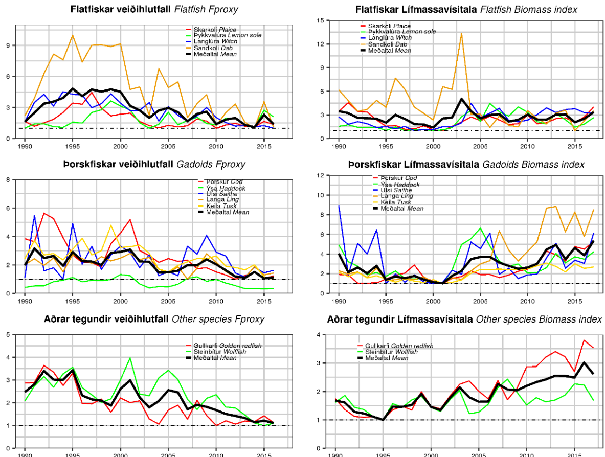
Mynd 4. Þróun F_{proxy} (afli/lífmassavísitala) og lífmassavísitala úr stofnmælingum, í hlutfalli við lægstu gildi sem sést hafa. ATH að línur sem sýna meðaltöl eru líka staðlaðar við lægsta gildi hvers meðaltals.
