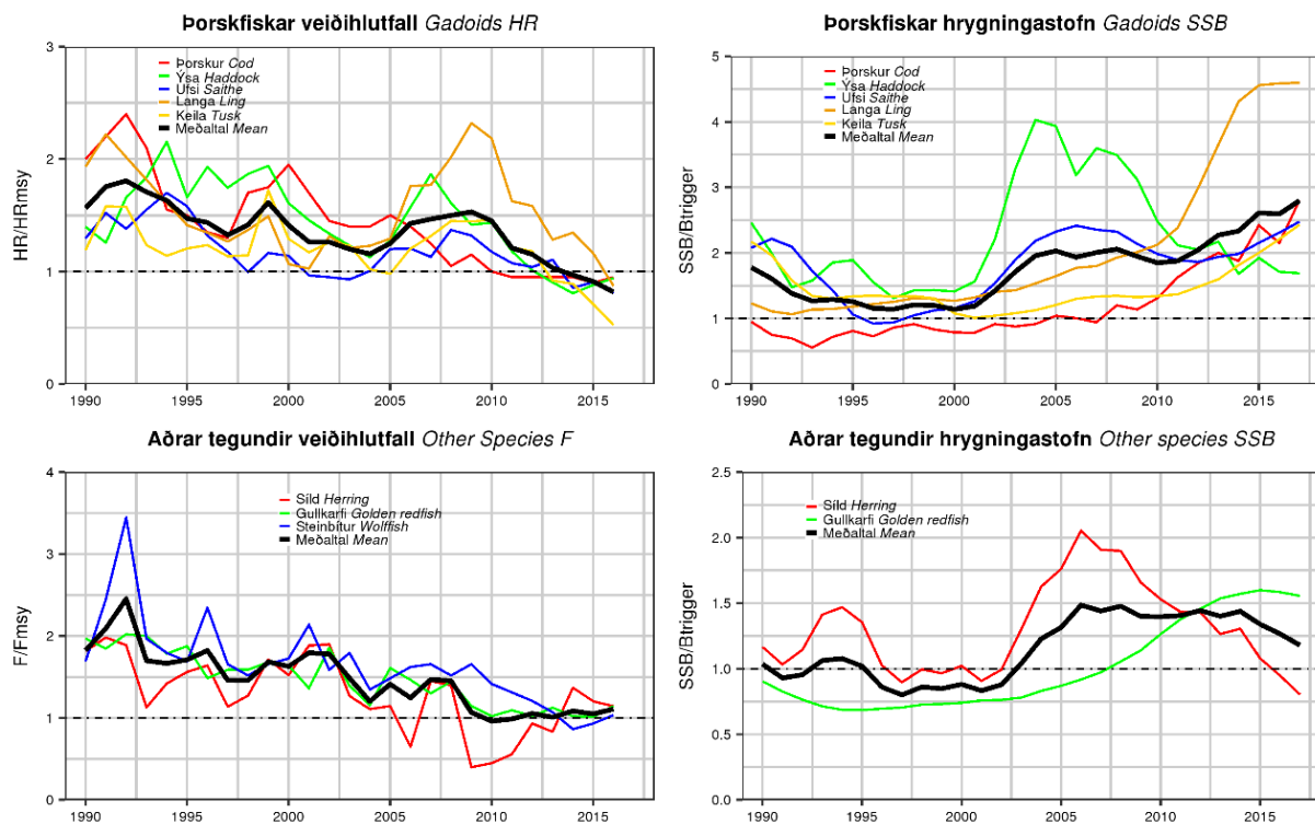
Mynd 3. Hlutfallslegt veiðiálág ( F/F_{MSY} eða HR/HR_{MSY} ) og hlutfallslegur hrygningarstofn ( SSB/B_{trigger} ) fyrir helstu tegundir á Íslandsmiðum.
