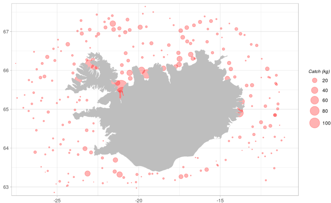
Figure 12. Long rough dab. Spatial distribution of long rough dab in 2016 in the autumn survey. Mynd 12. Skrápflúra. Útbreiðsla í stofnmælingu botnfiska að hausti árið 2016.
