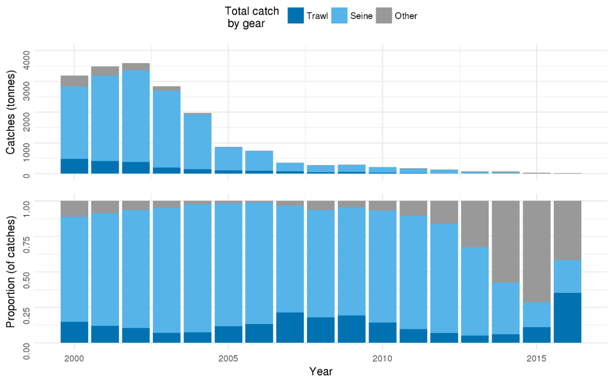
Figure 4. Long rough dab. Total catch (landings) by fishing gear since 2000. Mynd 4. Skrápflúra. Landaður afli eftir veiðarfærum frá 2000.
