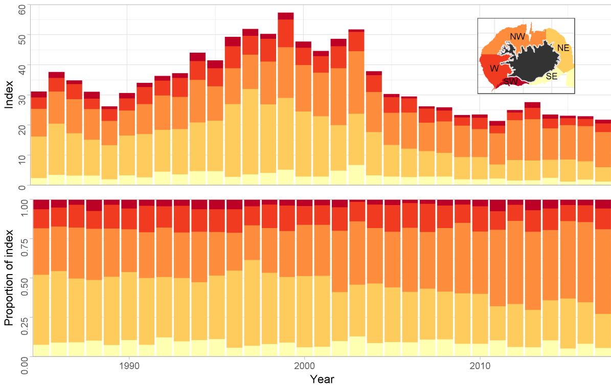
Figure 11. Long rough dab. Spatial distribution of biomass index from the spring survey in 1985-2017. Mynd 11. Skrápflúra. Dreifing lífmassavísitölu í stofnmælingu botnfiska að vori, árin 1985-2017.
