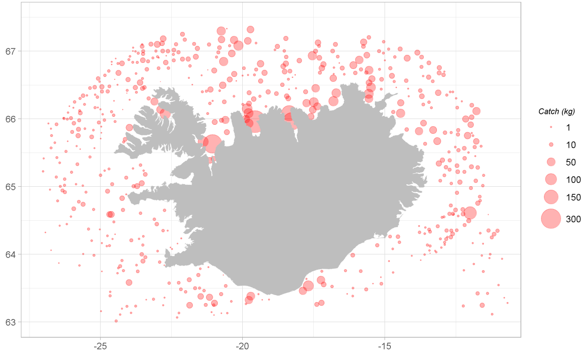
Figure 10. Long rough dab. Spatial distribution in the spring survey in 2017. Mynd 10. Skrápflúra. Útbreiðsla í stofnmælingu botnfiska að vori 2017.
