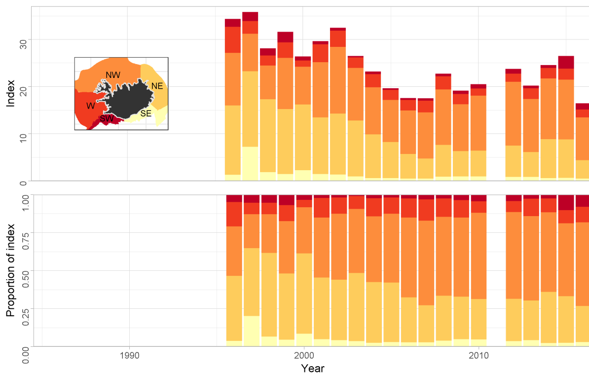
Figure 13. Long rough dab. Spatial distribution of biomass index from the autumn survey in 1996-2016. Mynd 13. Skrápflúra. Dreifing lífmassavísitölu í stofnmælingu botnfiska að hausti, árin 1996-2016.
