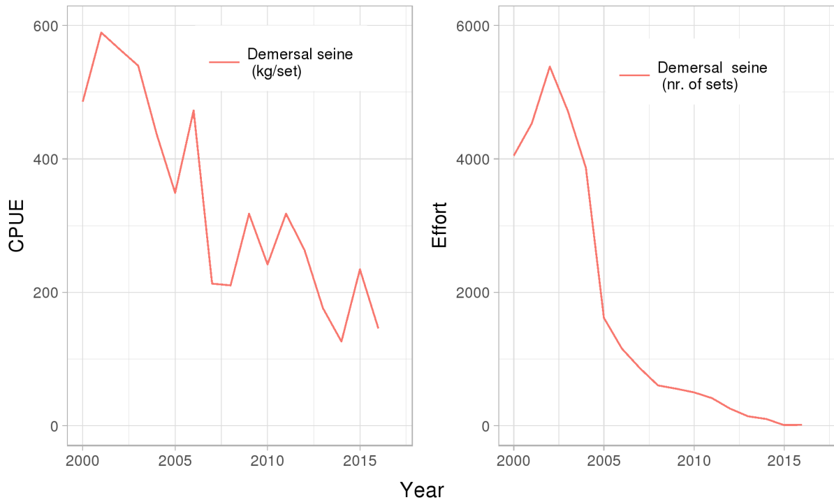
Figure 5. Long rough dab. Raw CPUE (left) and fishing effort (right) from demersal seine (kg/set or nr. of sets) Mynd 5. Skrápflúra. Afli á sóknareiningu (vinstri) og sókn (hægri) með dragnót (kg í kasti eða fjöldi kasta).
