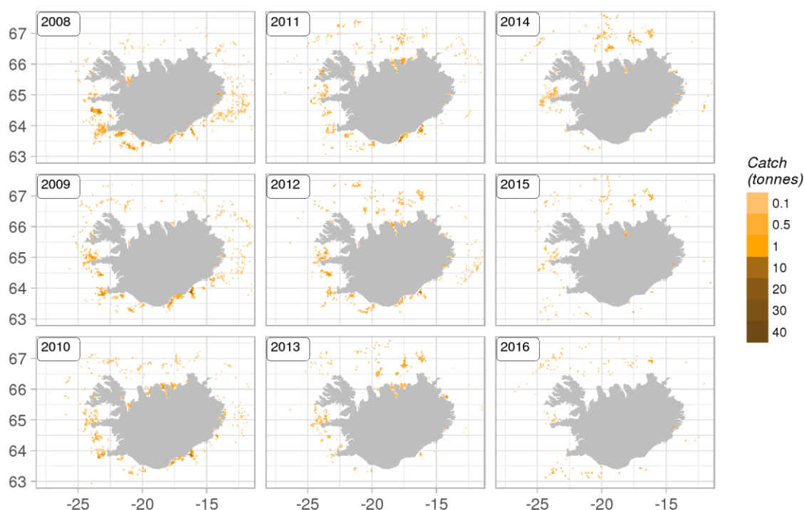
Figure 1. Long rough dab. Geographical distribution of the Icelandic fishery since 2008. Reported catch from logbooks. Mynd 1. Skrápflúra. Útbreiðsla veiða á Íslandsmiðum frá 2008 samkvæmt afladagbókum.
