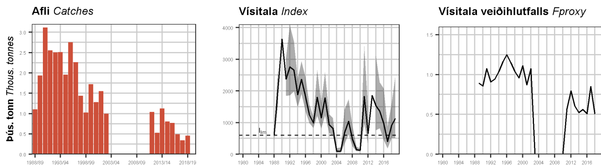
Rækja Ísafjarðardjúp. Afli, vísitala veiðistofns og vísitala veiðihlutfalls. Northern shrimp Ísafjarðardjúp. Catches, fishable biomass indices and F_{proxy} .
